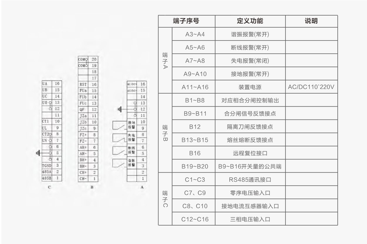
消弧柜控制器接线图和定义
