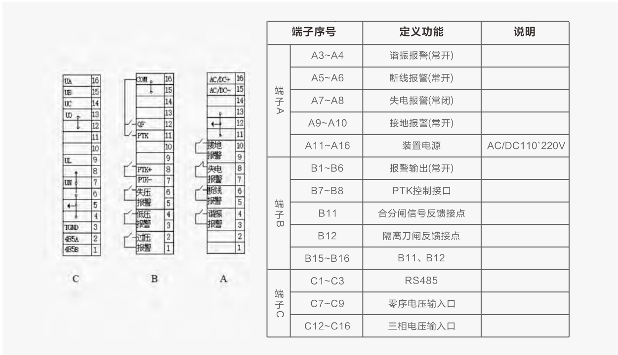
PTK控制器接线图和定义
