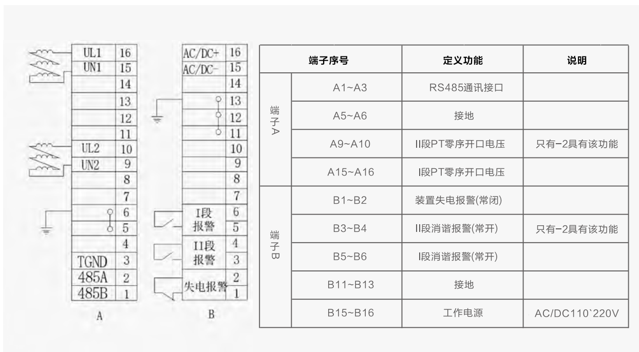
微机消谐装置接线图和定义
