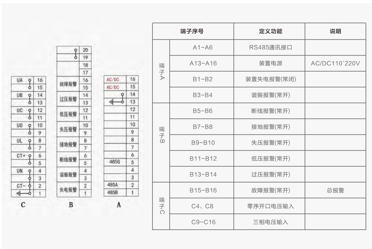
PT柜/抑制柜控制器接线图和定义
